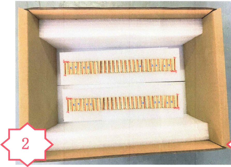
图二，将组件按图示装入箱内。一格 23 个，一层 两格，放 4 层，一箱一共 184 个
